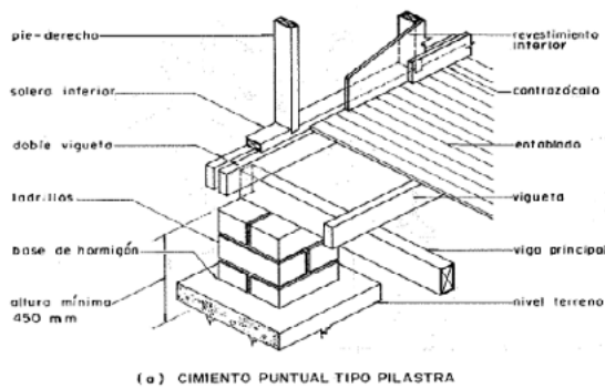
Cimiento tipo pilastra
