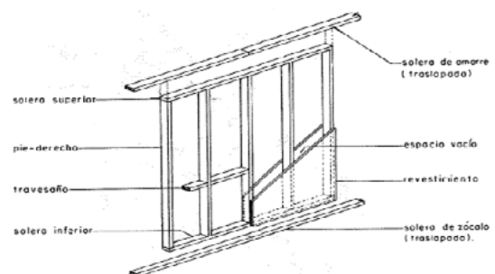
Figura 5.10 Muro entramado
